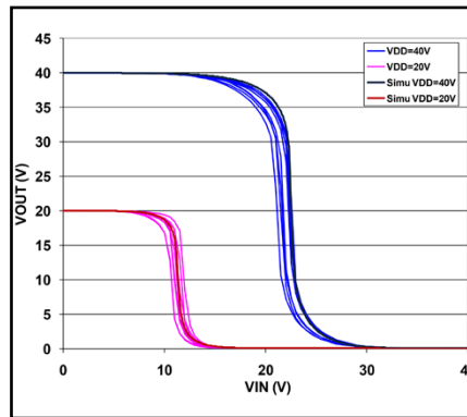
インバータにおける比較 (DCオペレーション)
