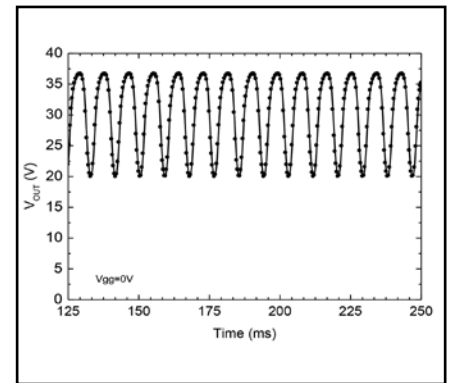
発振器における比較 (過渡オペレーション)
