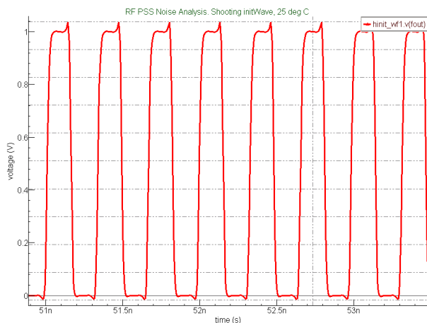
図4: ノードFOUTにおける波形
