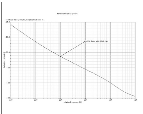
図9: 競合他社ベンチマークの位相ノイズ・プロット
