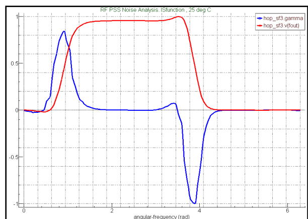
図5: ノードFOUTにおける正規化された波形および ISF (Impulse sensitivity function)
