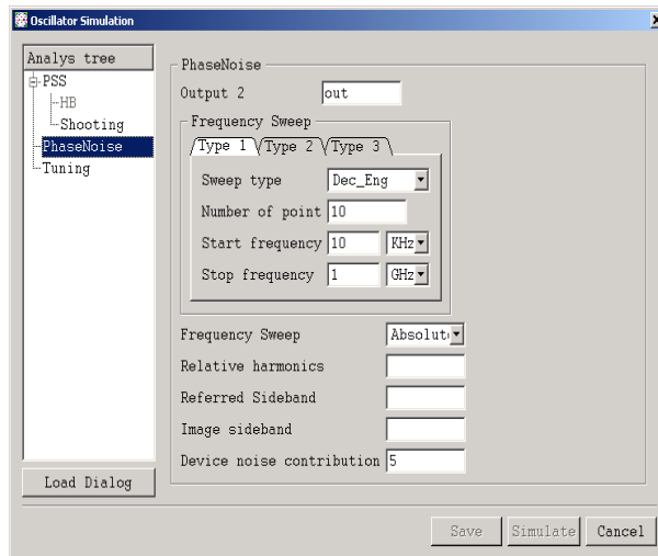
図6: 位相ノイズのダイアログ
