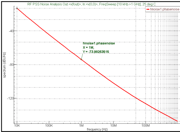
図8: SmartSpiceRFの位相ノイズ・プロット
