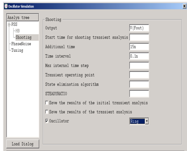
図3: シューティング法のダイアログ
