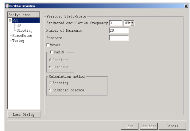
図1: PSS解析のダイアログ
